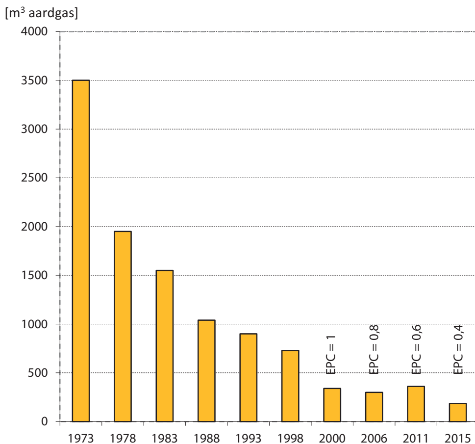
Afb. 1.10 Jaarlijks energieverbruik in m 3 aardgas voor ruimteverwarming (excl. elektriciteit voor CV-pomp) van een gemiddelde nieuwbouwwijzigingswoning gespecificeerd naar bouwjaar. Het gaat hierbij om berekende waarden. De waarden voor 2011 en 2015 zijn berekend met NEN 7120 (EPG). (Bron: [13] en referentiewoningen van RVO vanaf 1993)
