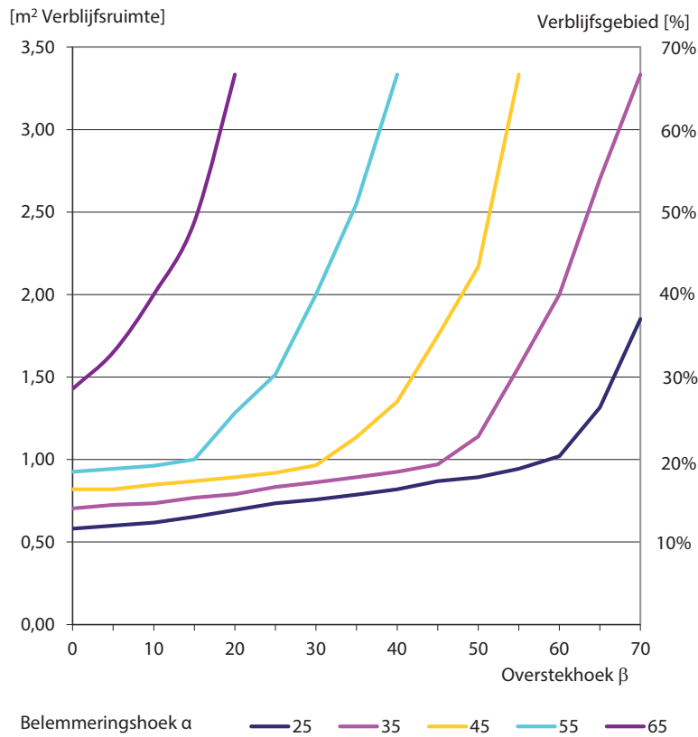
Afb. 4.24 Werkelijke daglichtopeningen om te voldoen aan de vereiste equivalente daglichtopening voor een verblijfsruimte (links m 2 ) en verblijfsgebied (rechts % vloeroppervlak) bij verschillende belemmeringshoeken \alpha en overstekhoeken \beta . Berekend volgens NEN 2057 [82].
