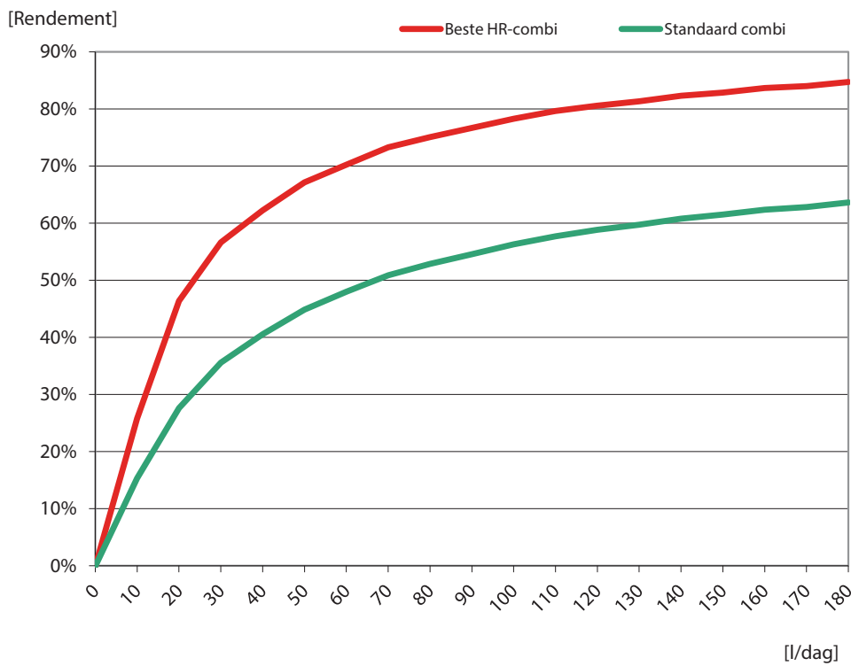
Afb. 9.9 Het gebruikrendement is afhankelijk van de vraag. Het gebruik van een huishouden ligt tussen 60 en 180 liter per dag; per persoon gebruikt men globaal 40 liter heetwater per dag
