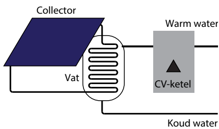
Afb. 9.16 De standaard zonneboiler. Er zijn zowel staande als liggende voorraadvaten verkrijgbaar
